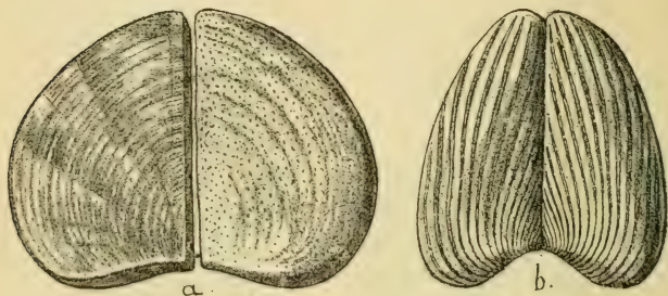
Fig. 326.
